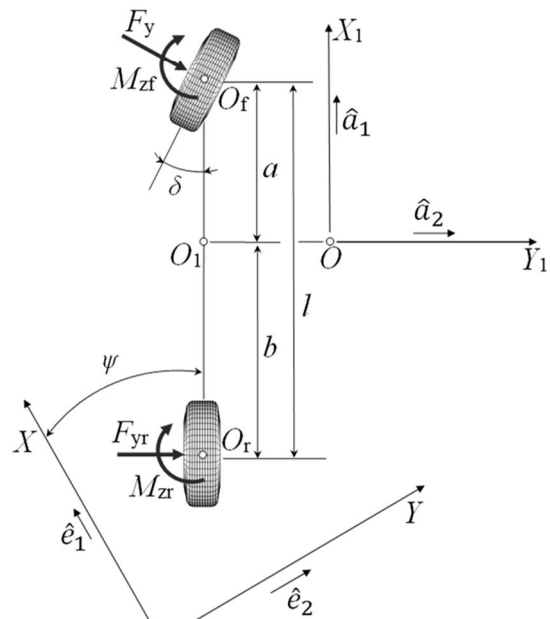
شکل 2 نمای صفحه ای عقب (بالا) و نمای صفحه ای بالا (پایین) خودرو صلب در زمان حرکت روی دو چرخ
