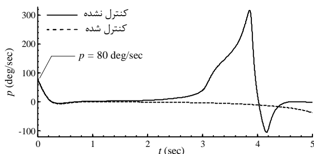
شکل 17 تغییرات نرخ زاویه رول خودرو با اعمال گشتاور اصلاحی در مانور کلایم اوور
