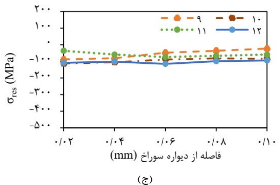
شکل ۷) توزیع تنش‌های پسماند نسبت به فاصله از سطح سوراخ در فرایندهای الف) سوراخ‌کاری معمولی ب) سوراخ‌کاری چندمرحله‌ای ج) فرزکاری ماریچ
