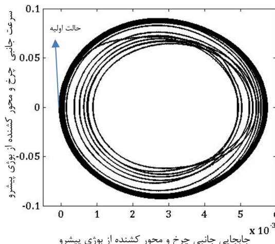
شکل 6 سرعت جانبی چرخ و محور کشنده از بوژی پیشرو (\dot{y}_{w1}) برحسب جابجایی جانبی آن (y_{w1}) (برای سرعت 317/5 کیلومتر بر ساعت)
