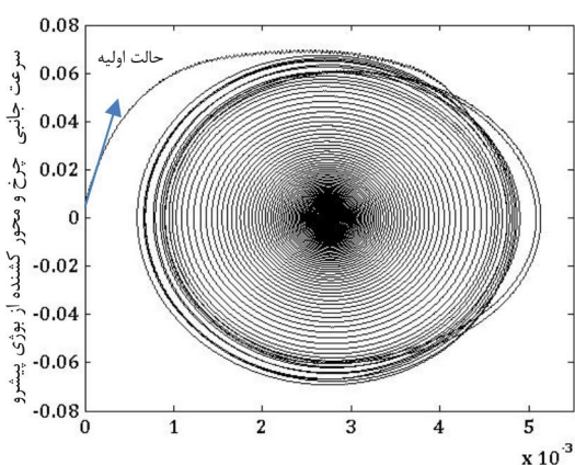
شکل 4 سرعت جانبی چرخ و محور کشته از بوژی پیشرو ( \dot{y}_{w11} ) بر حسب جابجایی جانبی آن ( y_{w11} ) (برای سرعت 312 کیلومتر بر ساعت)
