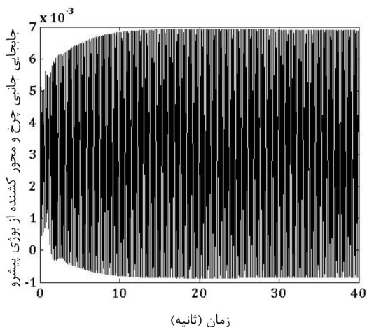
شکل 7 جابجایی جانبی چرخ و محور کشنده از بوژی پیشرو بر حسب زمان (ثانیه) (برای سرعت 320 کیلومتر بر ساعت)
