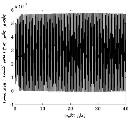
شکل 5 جابجایی جانبی چرخ و محور کشته از بوژی پیشرو بر حسب زمان (برای سرعت 317/5 کیلومتر بر ساعت)
