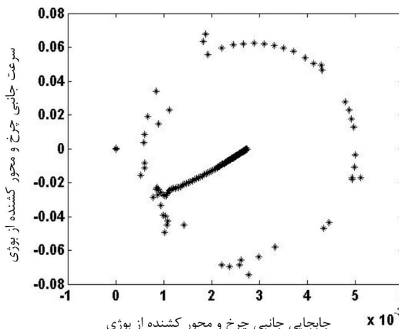
شکل 13 نگاشت پونکاره سرعت جانبی چرخ و محور کشنده از بوژی پیشرو برحسب جابجایی جانبی آن (برای سرعت 317/5 کیلومتر بر ساعت)
