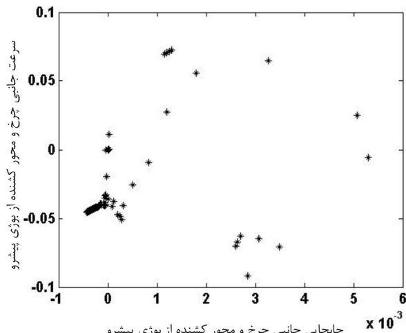
شکل 14 نگاشت پونکاره سرعت جانبی چرخ و محور کشنده از بوژی پیشرو جابجایی جانبی آن (برای سرعت 320 کیلومتر بر ساعت)
