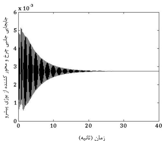
شکل 3 جابجایی جانبی چرخ و محور کشته از بوژی پیشرو بر حسب زمان (برای سرعت 312 کیلومتر بر ساعت)
