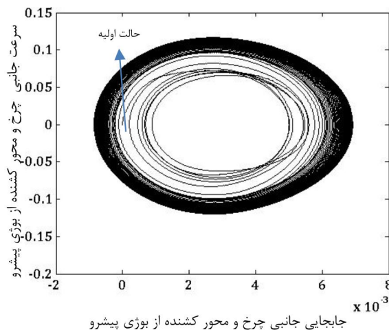
شکل 8 سرعت جانبی چرخ و محور کشنده از بوژی پیشرو (\dot{y}_{w1}) برحسب جابجایی جانبی آن (y_{w1}) (برای سرعت 320 کیلومتر بر ساعت)
