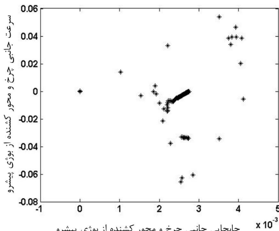
شکل 12 نگاشت پونکاره سرعت جانبی چرخ و محور کشنده از بوژی پیشرو برحسب جابجایی جانبی آن (برای سرعت 312 کیلومتر بر ساعت)
