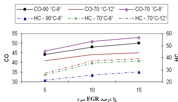
شکل ۷ تغییرات CO و HC با دمای خنک کاری و آوانس پاشش سوخت به ازای دردهای مختلف EGR
