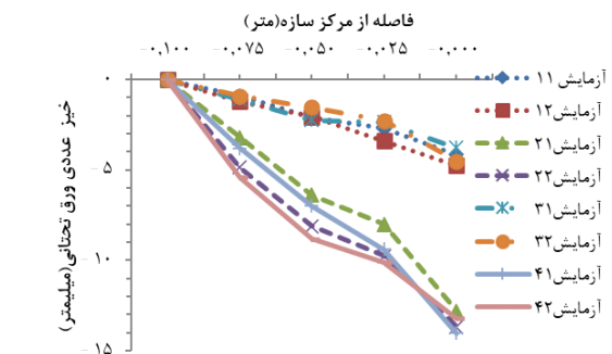
نمودار ۳) خیز ورق تحتانی بر حسب فاصله از مرکز سازه به روش عددی
