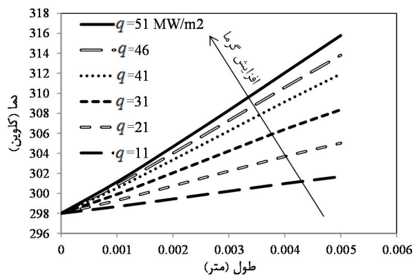
شکل 18 توزیع دمای سیال مایع در امتداد مینی کانال با شار گرمایی مختلفی
