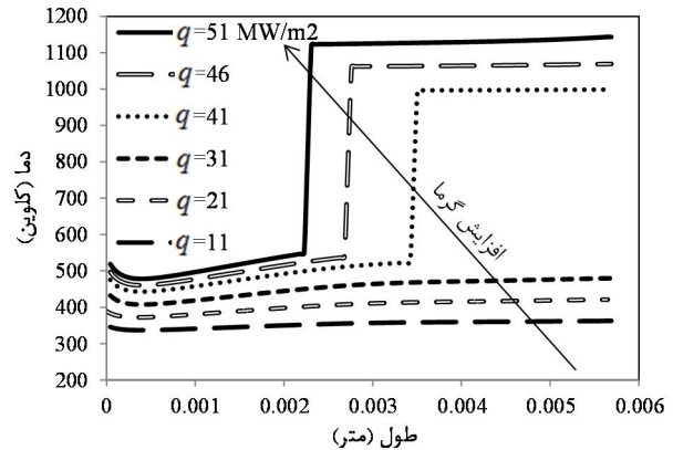
شکل 16 توزیع دمای دیواره در امتداد مینی کانال با شار گرمایی مختلفی
