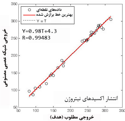
شکل ۱۵ آنالیز رگرسونی میان خروجی شبکه و خروجی مطلوب برای پیش‌بینی انتشار آلاینده‌های نیتروژن
