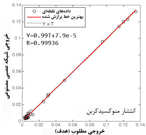
شکل ۱۴ آنالیز رگرسونی میان خروجی شبکه و خروجی مطلوب برای پیش‌بینی انتشار آلاینده منوکسید کربن
