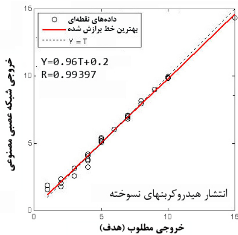
شکل ۱۶ آنالیز رگرسونی میان خروجی شبکه و خروجی مطلوب برای پیش‌بینی انتشار هیدروکربن‌های نسوخته
