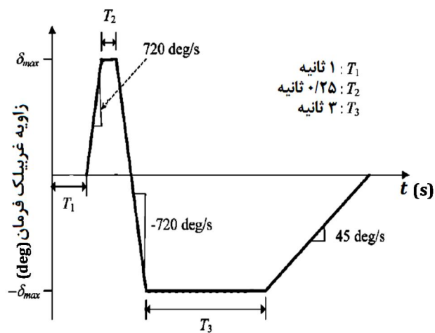
شکل 5 آزمون استاندارد قلاب ماهی [16]
