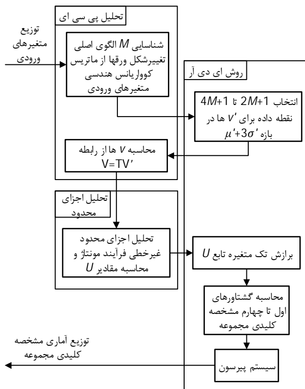
شکل 7 فرایند تحلیل تکرانسی سازه‌های ورق‌ی انعطاف‌پذیر
