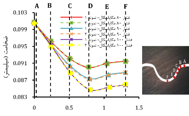
شکل ۳۸ منحنی توزیع ضخامت در راستای شیری
