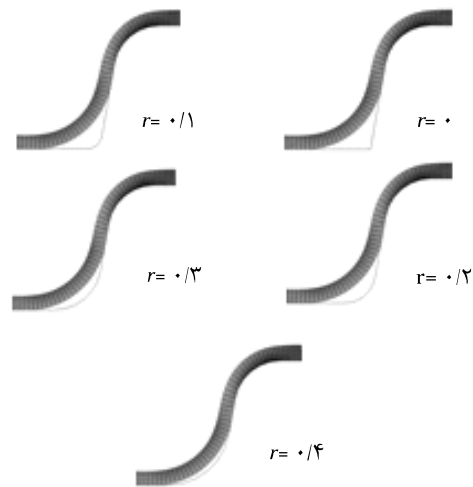
شکل ۳۳ نتایج شبیه‌سازی قالب‌هایی با شعاع فیلد خارجی R=0.3 mm
