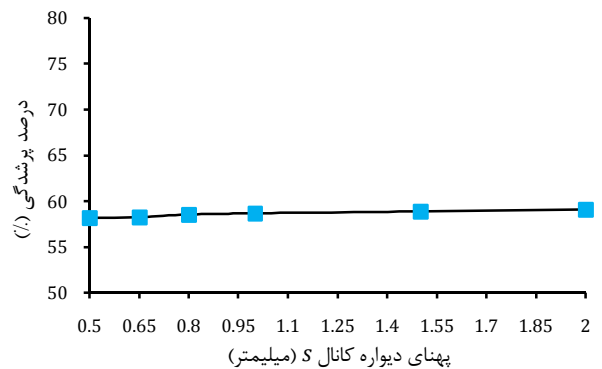
شکل ۱۸ مقایسه درصد پورندگی در پهنای دیواره کانال (s) مختلف
