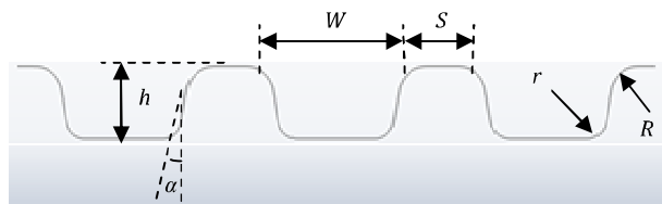
شکل ۳ طرح اولیه الگوی شیاری و نمایی از سطح مقطع آن
