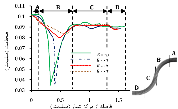
شکل ۳۱ منحنی توزیع ضخامت ورق شکل داده شده با قالب‌هایی با شعاع فیلت خارجی r=۰
