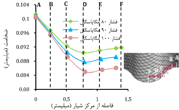
شکل ۳۶ منحنی توزیع ضخامت ورق شکل داده شده در راستای شیری
