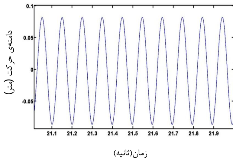
شکل 5 حرکت پیستون جابه‌جاگر در حالت پایدار
