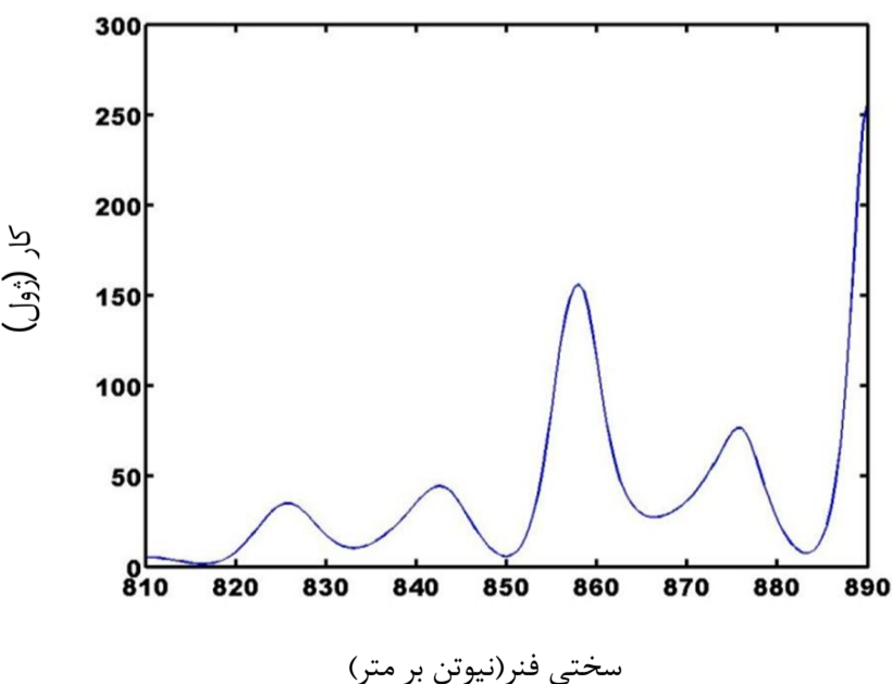
شکل 34 اثر افزایش سختی پیستون کار بر روی کار تولید شده در هر چرخه
