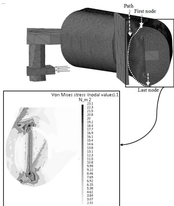
Fig. 5 stress distribution along the surface defined path شکل 5 توزیع تنش در پروتز و روکش بر اثر بارگذاری در طول مسیر تعیین شده
