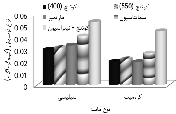
شکل 8 نرخ سایش فرسایشی فولاد AISI H13 با انواع ماسه ماهیچه در فشار پاشش 3 بار
