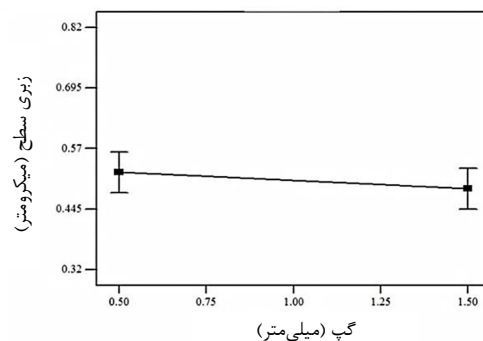
شکل ۱۳ تأثیر پارامتر ورودی گپ کاری بر خروجی فرآیند (زبری سطح)
