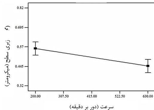
شکل ۱۲ تأثیر پارامتر ورودی سرعت دورانی برس ساینده بر خروجی فرآیند (زبری سطح)
