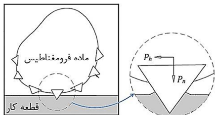
شکل ۱ شکل‌گیری ذرات ساینده [6]
