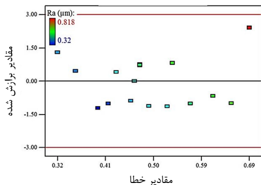
شکل ۴ نمودار خطا در برابر مقادیر برازش شده
