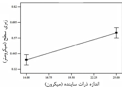
شکل ۶ تأثیر پارامتر ورودی مش ذرات ساینده بر خروجی فرآیند (زبری سطح)
