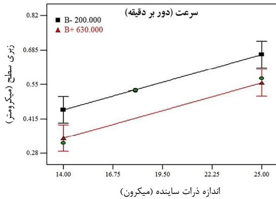
شکل ۹ تأثیر همزمان اندازه دانه و سرعت چرخش بر خروجی فرآیند (زبری سطح)
