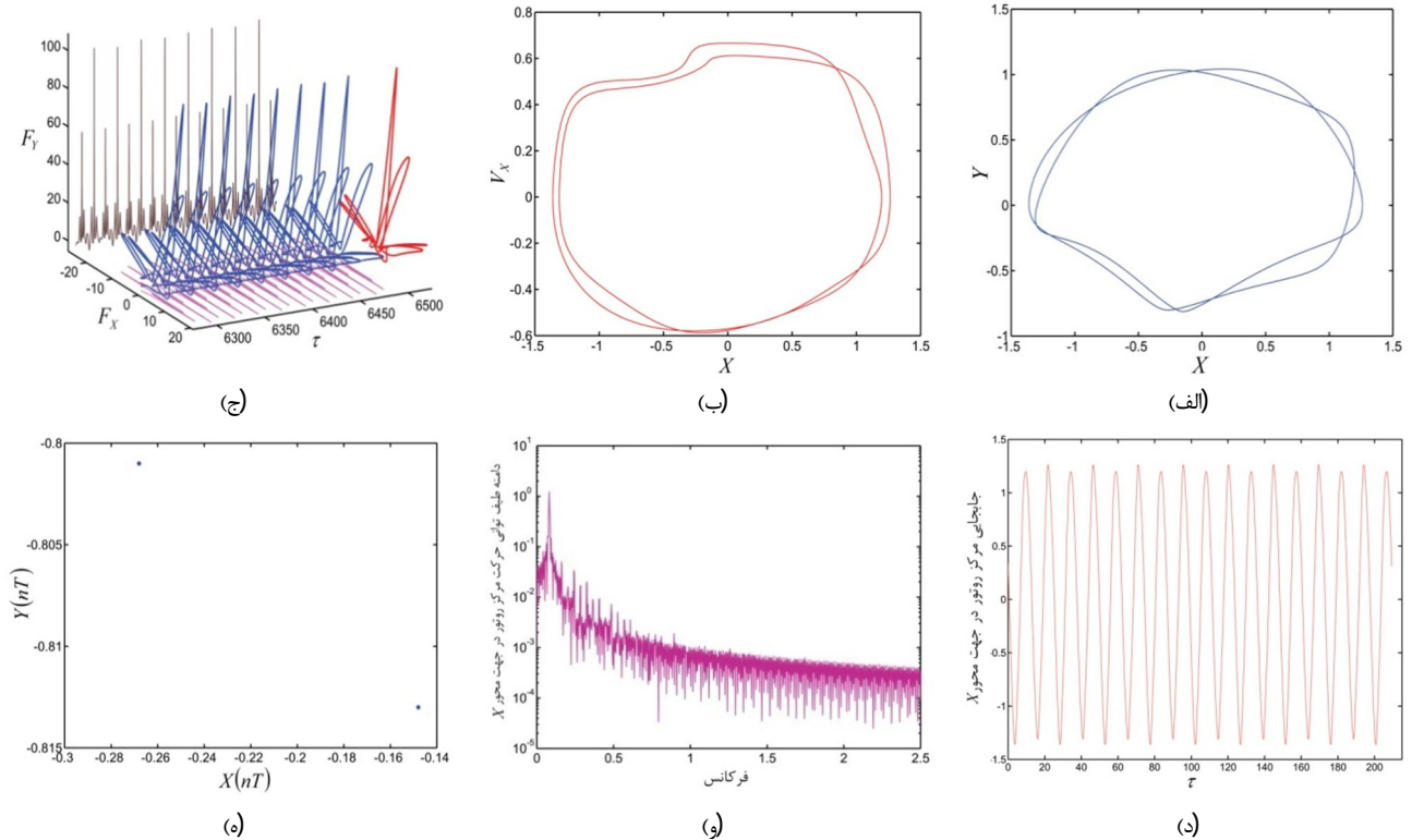
شکل 5 (الف) مسیر حرکت مرکز روتور (ب) تصویر فاز مرکز روتور (ج) مولفه‌های نیروی دینامیکی (د) سری زمانی حرکت روتور (و) طیف توانی جابجایی روتور (ه) نگاهت پوانکاره
