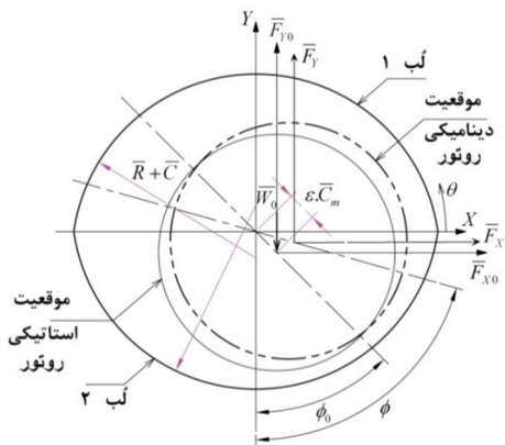
شکل 3 بارگذاری محور در شرایط دینامیکی یاتاقان ژورنال غیرمدور دو لب
