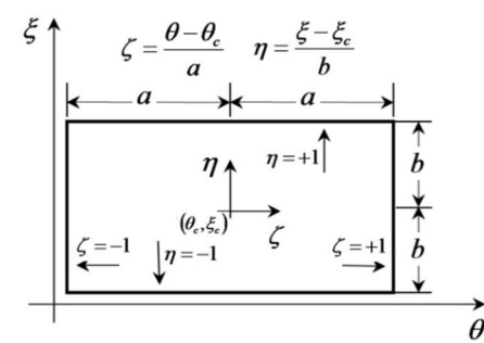
شکل 2 مختصات طبیعی (\eta, \zeta) المان مستطیلی
