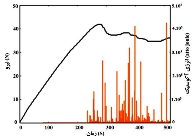
شکل ۲ نمودار انرژی آکوستیک-زمان
