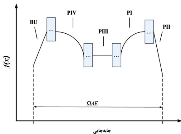
شکل ۳ توابع تشکیل دهنده تابع انرژی کرنشی SF
