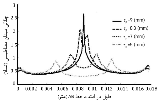
شکل 7 میدان مغناطیسی بر حسب طول دو قطب به ازاء ابعاد مختلف
