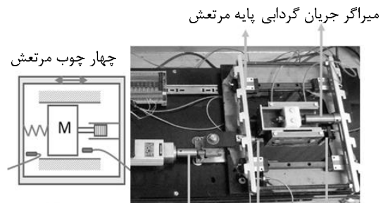
شکل 13 مجموعه آزمایشگاهی
