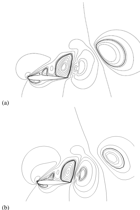
Fig. 7 v -velocity contours on the NACA0012, \alpha = 20^\circ , Re = 800 and t = 5 (a): Hafez et al [28] (b): Current study شکل 7 خطوط همتراز سرعت عمودی v هیدروفویل NACA0012، \alpha = 20^\circ ، Re = 800 و زمان t = 5 . (a): حافظ [28]؛ (b): مطالعه‌ی حاضر
