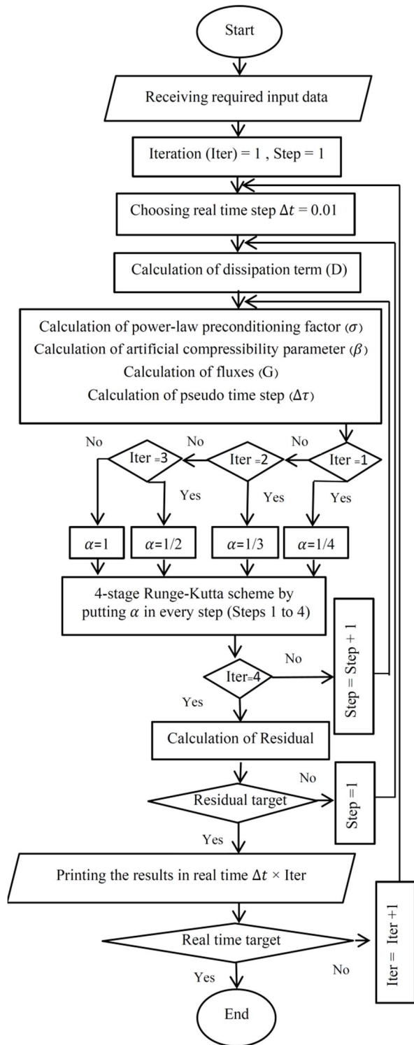
Fig. 1 The flowchart of the computational algorithm شکل 1 روندنمای الگوریتم محاسباتی
