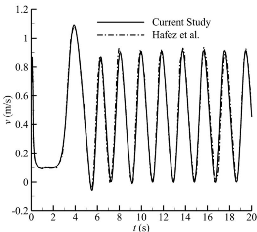
Fig. 4 Comparison of time variation of the v -velocity at x = 1.1 , y = 0.0 behind the NACA0012, \alpha = 20^\circ and Re = 800 [28] شکل 4 مقایسه تغییرات سرعت عمودی v در موقعیت x = 1.1 , y = 0.0 پشت هیدروفویل NACA0012 بر حسب زمان، \alpha = 20^\circ و Re = 800 [28]
