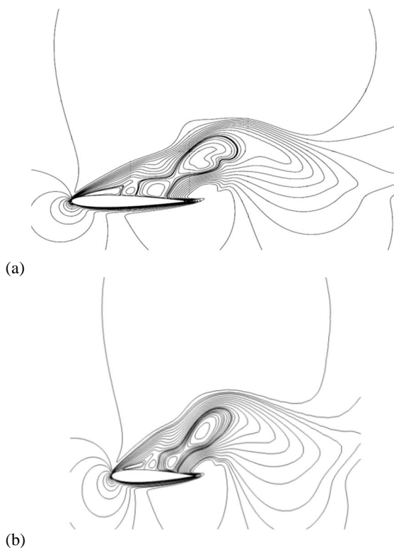
Fig. 8 u -velocity contours on the NACA0012, \alpha = 20^\circ , Re = 800 and time = 5 (a): Hafez et al [28] (b): Current study شکل 8 خطوط همتراز سرعت افقی u هیدروفویل NACA0012، \alpha = 20^\circ ، Re = 800 و زمان t = 5 . (a): حافظ [28]؛ (b): مطالعه‌ی حاضر
