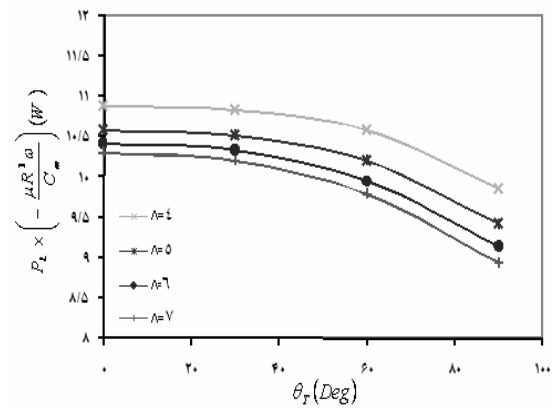
شکل ۱۲ اثر زاویه انحراف ( \theta_r ) بر افت انرژی ( P_L ) پاتاقان دو - لب
