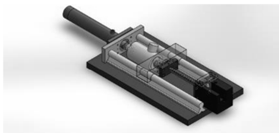
شکل ۸. مدل سه‌بعدی مکانیزم مورد استفاده در آزمایش‌ها
