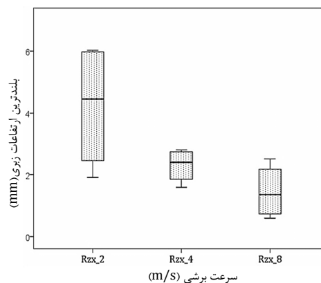
شکل ۱۰ نمودار جعبه‌ای میانگین زبری سطح میانگین بلندترین ارتفاعات زبری
