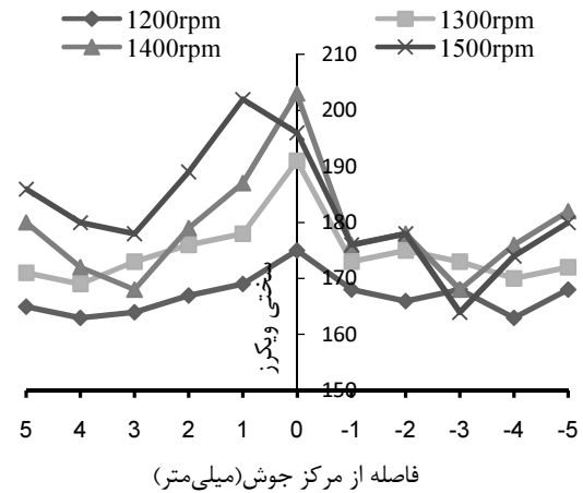
شکل ۹ تأثیر سرعت دورانی روی ریز سختی
