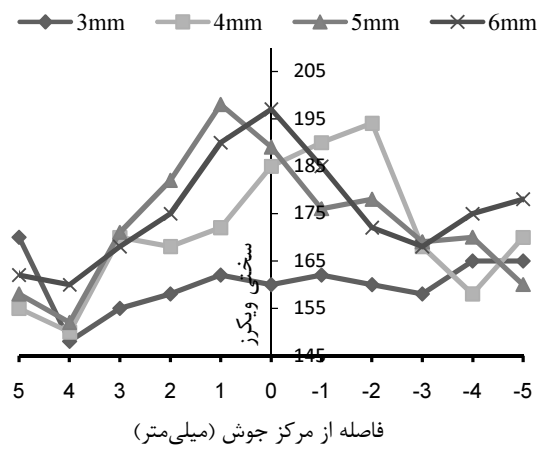
شکل ۱۲ تأثیر قطر پین روی ریز سختی
