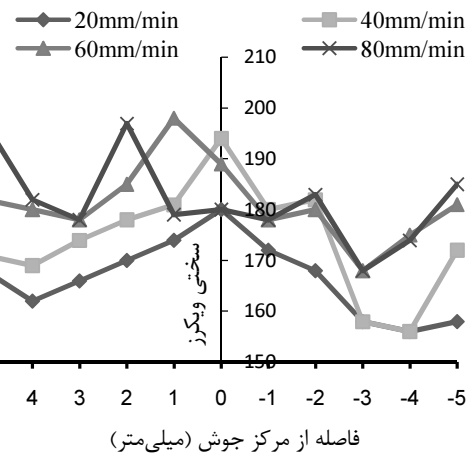
شکل ۱۰ تأثیر سرعت جوش کاری روی ریز سختی
