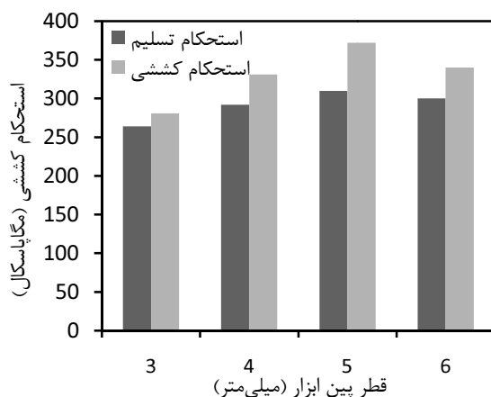
شکل ۷ تأثیر قطر بین روی خواص مکانیکی
