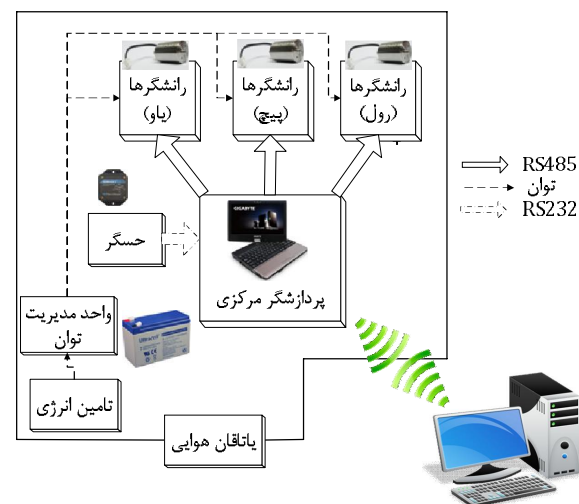
شکل 6 معماری سیستم شبیه‌ساز دینامیک وضعیت 1001
