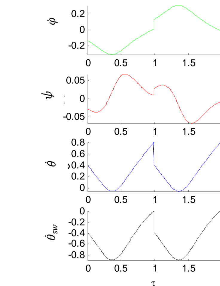
شکل 17 تغییر سرعت‌های تعمیم‌یافته ربات حین یک گام (دو قدم متوالی). محورهای افقی نمایش‌گر زمان بی‌بعد \tau هستند.
