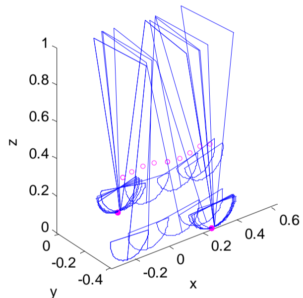
شکل 5 مجموعه تصاویر کنترل راه رفتن پایدار مجانبی روی سطح صاف حین یک گام (دو قدم متوالی). مرکز جرم کل ربات در هر لحظه با علامت دایره «o» مشخص شده است.
