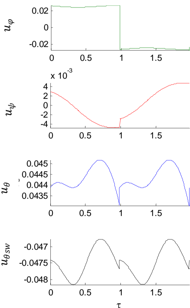
شکل 19 تغییر ورودی‌های کنترلی حین یک گام پریودیک (دو قدم متوالی)
