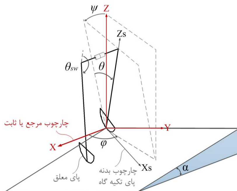
شکل 1 مدل پرگاری سه‌بعدی با عرض غیرصفر و کف پای منحنی
