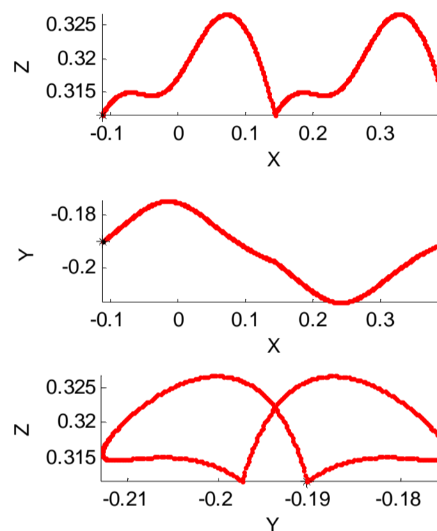
شکل 10 نمودار تغییر موقعیت مرکز جرم ربات حین یک گام در صفحات مختلف. موقعیت اولیه با علامت "*" مشخص شده است.
