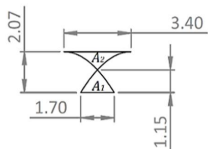
شکل 17 هندسه‌ی ناحیه‌ی هم‌پوشانی A_1 و ناحیه انباشت فلز A_2 برای مهره‌جوش بهینه (ابعاد به mm)
