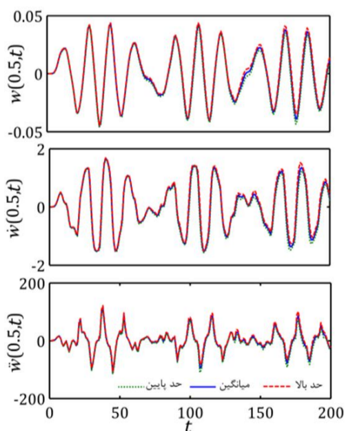
شکل 14 پاسخ‌های دینامیکی لوله حامل جریان چندفازی براساس مدل غیرخطی به‌ازای U = 1 و A = 5
