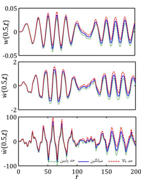
شکل 13 پاسخ‌های دینامیکی لوله حامل جریان چندفازی براساس مدل غیرخطی به‌ازای A = 3 و U = 1
