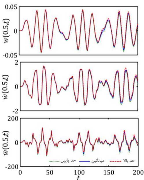
شکل 14 پاسخ‌های دینامیکی لوله حامل جریان چندفازی براساس مدل غیرخطی به‌ازای A = 5 و U = 1
