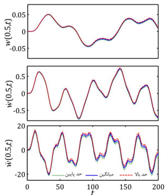
شکل 11 پاسخ‌های دینامیکی لوله حامل جریان چندفازی براساس مدل خطی به‌ازای U = 1 و A = 5
