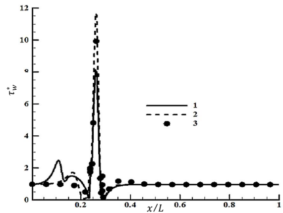
Fig. 7 WSS variation along the stenosis as the function of RBC location شکل 7 تغییرات تنش برشی بر اساس محل گلبول قرمز در طول گرفتگی
