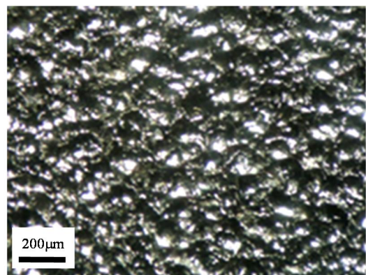
شکل 12 بافت سطحی نمونه‌های مسی پس از قرارگیری تحت تخلیه‌ی الکتریکی
