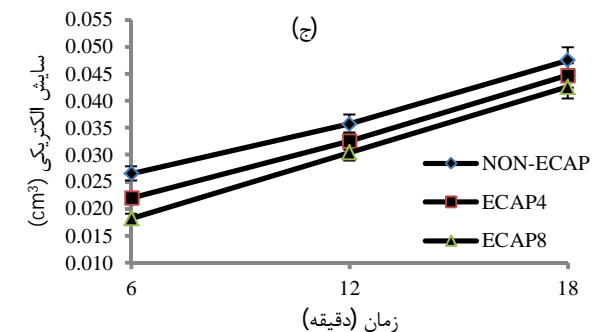
شکل 11 سایش الکتریکی نمونه‌های مسی ECAP4، ECAP8 و نمونه‌ی اولیه بر حسب زمان به ترتیب در شدت جریان‌های - (الف) 5 (ب) 10 و (ج) 15 آمپر
