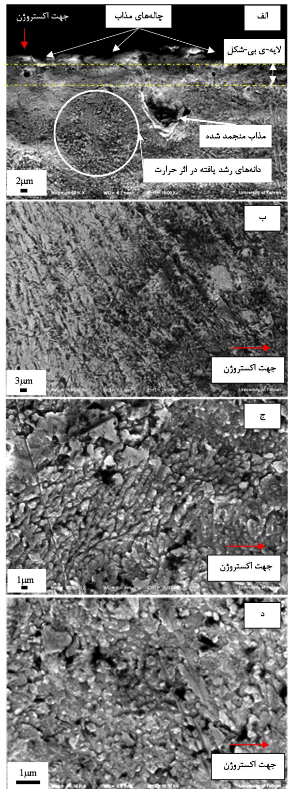
شکل 14 تصویر FE-SEM از ریز ساختار زیر لایه‌ی عمق - الف (60μm ب) 200μm ج (400μm د) 900μm
