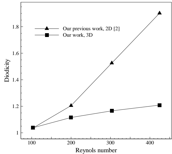
Fig. 6. Diodicity as Reynolds number in steady 2D and 3D simulations شکل 6 نمودار یکسوکندگی بر حسب عدد رینولدز در شبیه‌سازی دائم دوبعدی و سه‌بعدی
