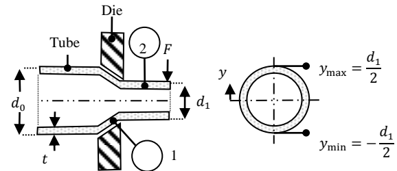
Fig. 2 Parameters of bent tube
