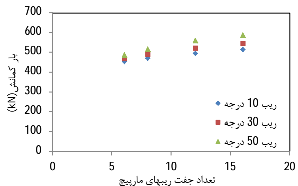
شکل 11 نمودار تغییرات بار کمانش بر حسب تعداد جفت ریب‌های مارپیچ به ازای زوایای مختلف ریب مارپیچ
