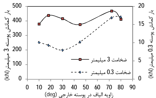
شکل 10 نمودار تغییرات بار کمانش بر حسب زاویه الیاف در پوسته خارجی برای 2 ضخامت مختلف
