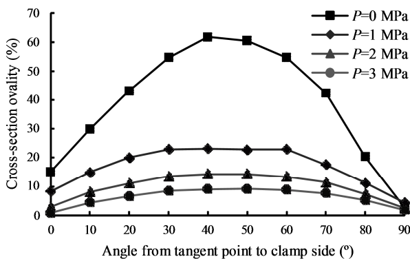
Fig. 17 The effect of internal pressure on the cross section distortion شکل 17 اثر فشار داخلی روی اعوجاج سطح مقطع لوله خم کاری شده
