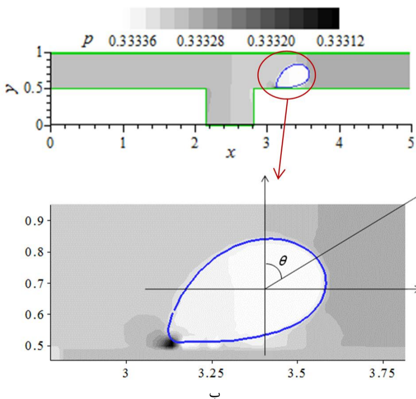
شکل 11 نمودار فشار نقاط لاگرانژی بر حسب زاویه (الف) و کانتورهای فشار سیال (ب) در زمان t=3/5
