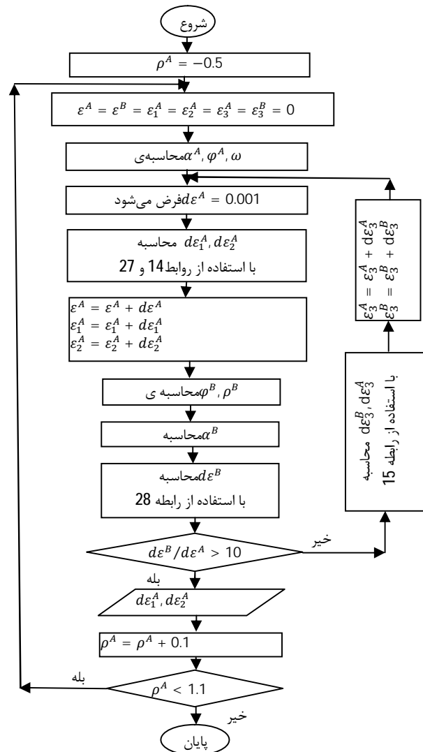
شکل 2 فلوچارت جهت تعیین کرنش‌های حدی براساس مدل MK
