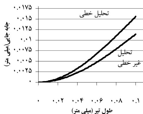
شکل ۹ تفاوت تحلیل خطی و غیرخطی در محاسبه جابه‌جایی انتهای آزاد تیر کامپوزیت پیزوالکتریک
