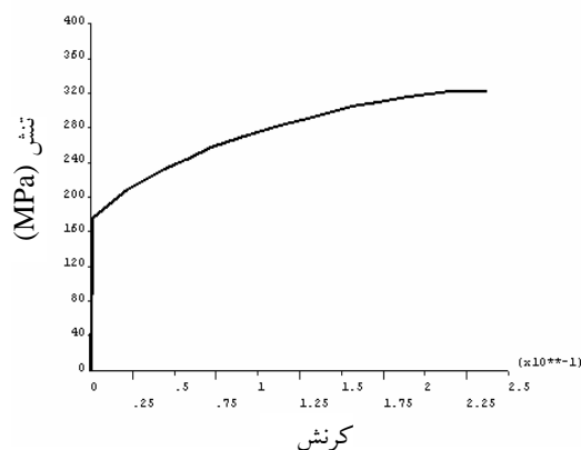
شکل ۵ منحنی تنش - کرنش حقیقی
