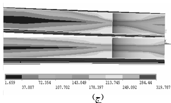
شکل ۹ کانتور تنش ون - مایز (الف) بارگذاری ۱۰۰۰ نیوتن در ناحیه اطراف نقطه جوش چهارم و در ورق پایه (ب) بارگذاری ۴۵۰۰ نیوتن در ناگت جوش (ج) ناگت جوش در نزدیکترین نقطه جوش
