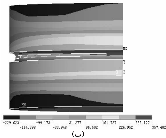
شکل ۱۰ (الف) \sigma_{11} برای بارگذاری ۱۰۰۰ نیوتن در نمونه با ۷ نقطه جوش (ب) تنش \sigma_x در ناگت جوش تحت بارگذاری ۴۵۰۰ نیوتن
