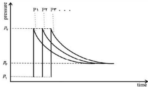
شکل ۴ شبیه‌سازی موج انفجار به صورت فشار متحرک
