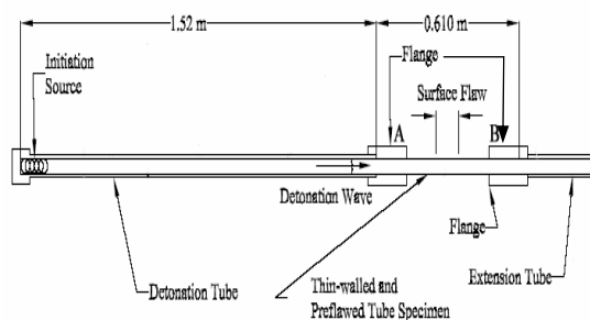
شکل ۳ لوله انفجار [۱]
