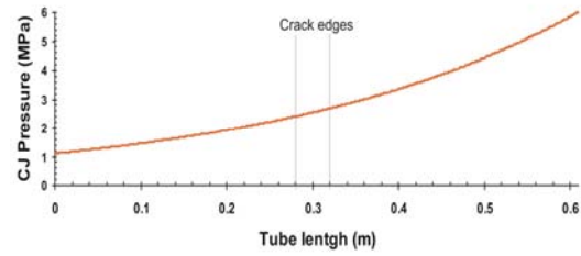
شکل ۱۴ توزیع فشار در راستای طول لوله زمانی که پیشانی موج انفجار به انتهای لوله می‌رسد
