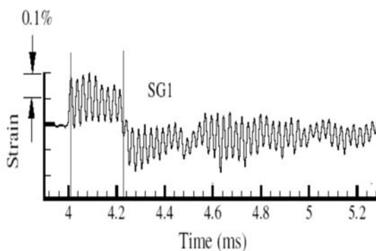
شکل ۱۰ تاریخچه کرنش مربوط به آزمایش شماره ۳۰ [۱]
