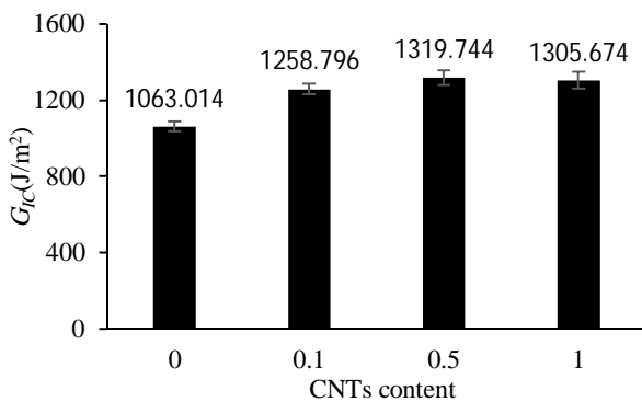
Fig. 15 The crack propagation mode I fracture toughness of nanocomposite calculated by compliance calibration method شکل 15 چقرمگی گسترش ترک مود اول شکست نانوکامپوزیت با روش کالیبراسیون نرمی
