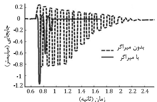
شکل 17 مقایسه نمودار پاسخ زمانی ارتعاشات آزاد میراگر با حالت بدون میرایی
