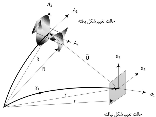
شکل 1 قالب‌بندی تغییر شکل تیر
