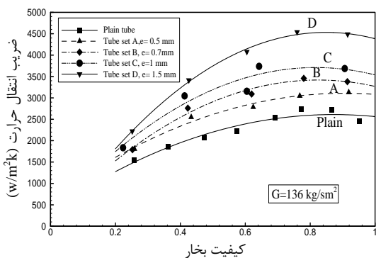
شکل ۷ تغییرات ضریب انتقال حرارت با تغییر کیفیت بخار برای لوله صاف و لوله‌های مجهز به سیم‌پیچ با گام ۱۰mm و در سرعت جرمی 136 \text{ kg/sm}^2
