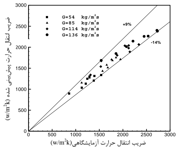
شکل ۳ مقایسه نتایج آزمایشگاهی لوله صاف با رابطه جانگر و وینرتون (رابطه ۸)
