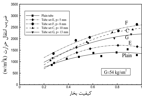
شکل ۸ تغییرات ضریب انتقال حرارت با تغییر کیفیت بخار برای لوله صاف و لوله‌های مجهز به سیم‌پیچ با قطر سیم ۱mm و در سرعت جرمی 54 \text{ kg/sm}^2
