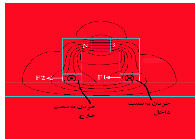
شکل 4 چگالی شار مغناطیسی و جهت نیروها
