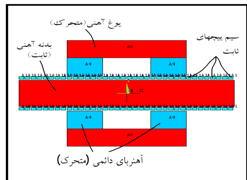
شکل 9 طرحواره دو بُعدی از طرح ارائه شده
