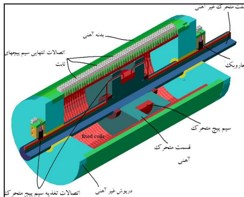
شکل 7 موتور لوله ای خطی با استفاده از سیم پیچ تحریک
