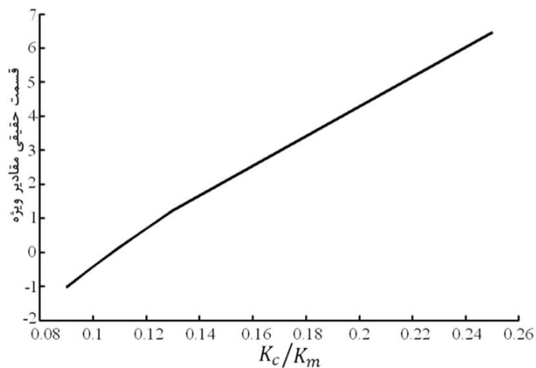
شکل 5 تغییر قسمت حقیقی مقادیر ویژه مربوط به ماتریس ریشه معادله (18)
