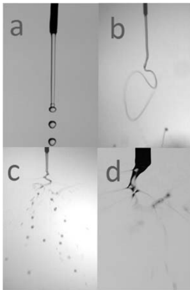
Fig. 16 The other modes, Flowrate= 250 ml/h, (a): Simple jet, Voltage= 3.92kV, (2): Oscillating simple jet, Voltage= 6.01kV, (c) Ramified jet, Voltage= 9.66kV, Random spray, Voltage= 12.81kV. شکل 16 سایر حالت‌های پاشش، دبی سیال 250 ml/h، (a): جت ساده، ولتاژ اعمالی 3.92kV، (b): جت ساده نوسانی، ولتاژ اعمالی 6.01kV، (c): جت منشعب، ولتاژ اعمالی 9.66kV، (d): پاشش تصادفی، ولتاژ اعمالی 12.81kV.
