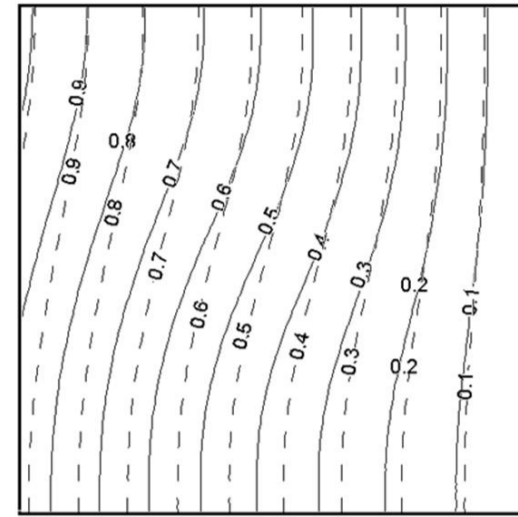
شکل 10 کانتورهای خطوط همدمای دو هارتمن مختلف 0 (خط چین) و 10 (خط ممتد) در عدد رایلی 10^3
