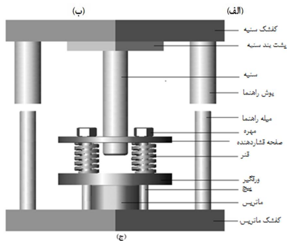
شکل 2 الف- دستگاه آزمایش اونیورسال (DMG) ب- مجموعه قالب استفاده شده در آزمایش‌های تجربی ج- شماتیک قالب کشش عمیق
