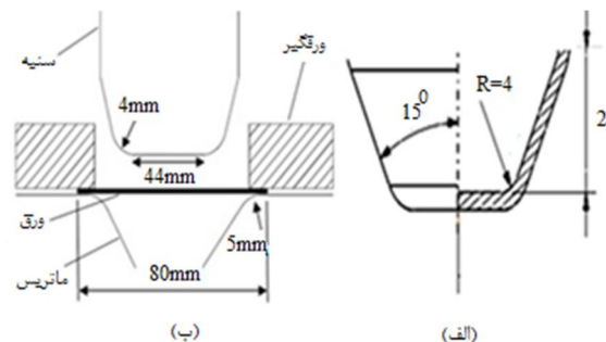
شکل 3 الف- هندسه قطعه ب- شماتیک قالب استفاده شده در این پژوهش
