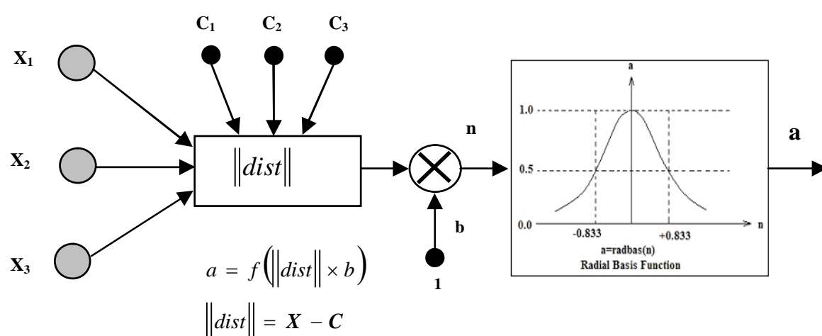
Fig. 4 Radial basis neuron.
