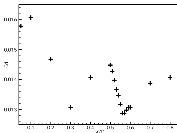
شکل 15 نمودار ضریب پسی ایرفویل با قرارگیری برآمدگی در فواصل مختلف
