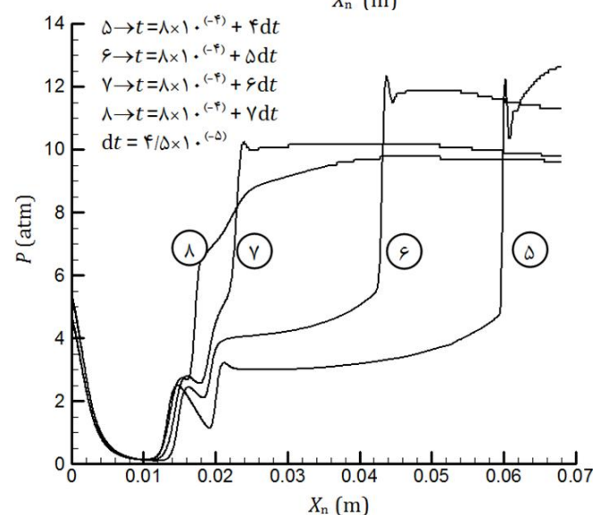
شکل 15 توزیع فشار در خط مرکزی در زمان‌های مختلف سیکل ورود و خروج موج در بخش اول جریان (بازه زمانی بین 8 \times 10^{-4} تا 11 \times 10^{-4} )
