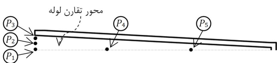
شکل 8 نمایی از محل قرار گرفتن نقاط نمونه درون لوله تشدید
