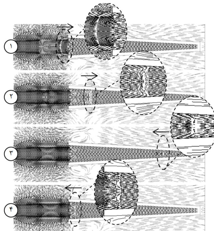
شکل 12 آرایش خطوط جریان در جت ورودی و درون لوله و نمایش جابجایی امواج تراکمی در زمان تعویض رژیم از سیکل تخلیه به سیکل پر شدن
