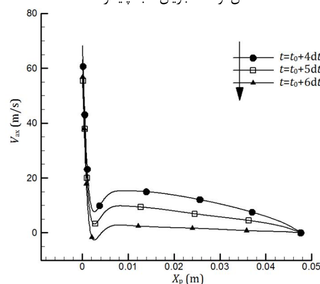
شکل 22 تغییرات سرعت محوری در خط مرکزی جریان در بخش دوم نیم سیکل پر شدن لوله - جریان شبه پایدار
