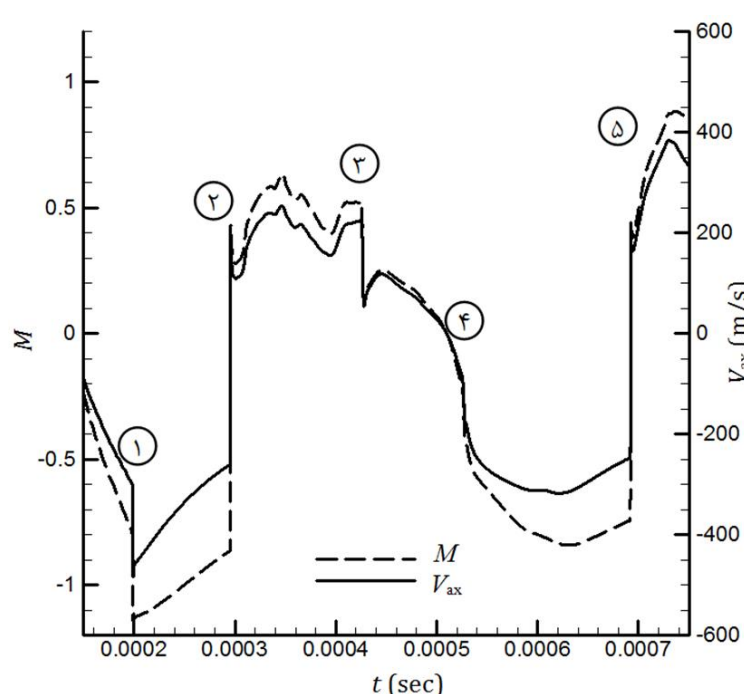
شکل 10 روند تغییرات سرعت محوری و عدد ماخ جریان در نقطه P_4
