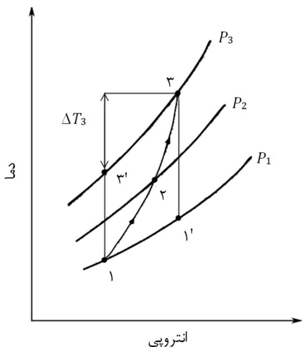
شکل 2 نمودار دما - انترپوی در فرآیند درونی لوله تشدید و خطوط فشار ثابت [9]
