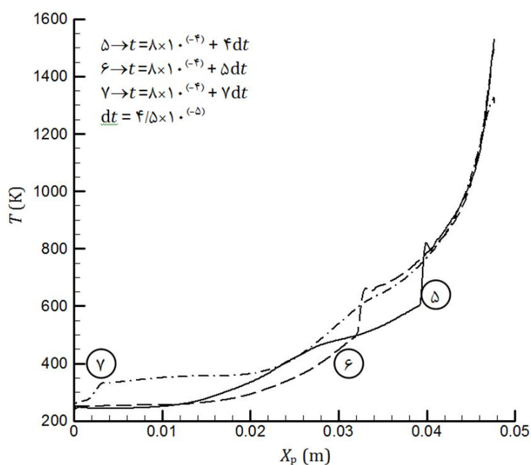
شکل 16 توزیع دما در خط مرکزی در زمان‌های مختلف سیکل ورود و خروج موج در بخش اول جریان (بازه زمانی بین 8 \times 10^{-4} تا 11 \times 10^{-4} )
