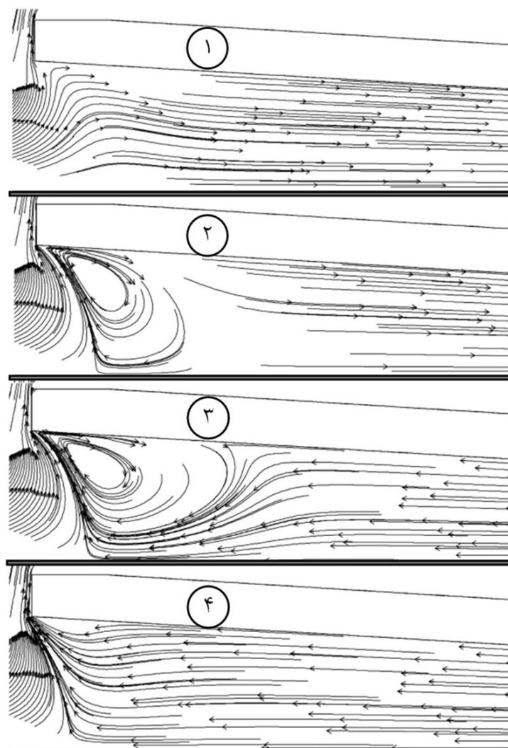
شکل 17 آرایش خطوط جریان در مقطع ورودی نیم‌لوله در طول یک دوره زمانی ورود و خروج جریان در قسمت شبه پایدار حل (بخش دوم)
